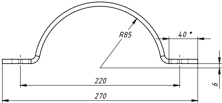
Поз.2 (Полухомут) развертка
