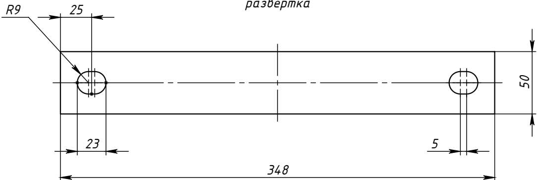
Поз.2 (Полухомут) развертка
